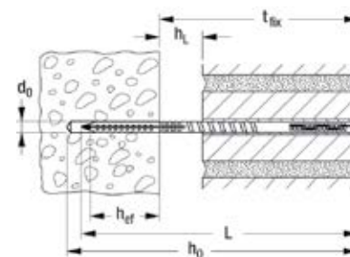
Механический ремонтный анкер VBS-M
